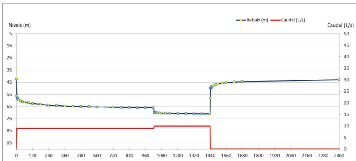
Figura 5.29 – Ensaio de caudal RAQ023 (RA1 - LSM1) Fonte: EIA do Projeto Agroflorestal LSM
