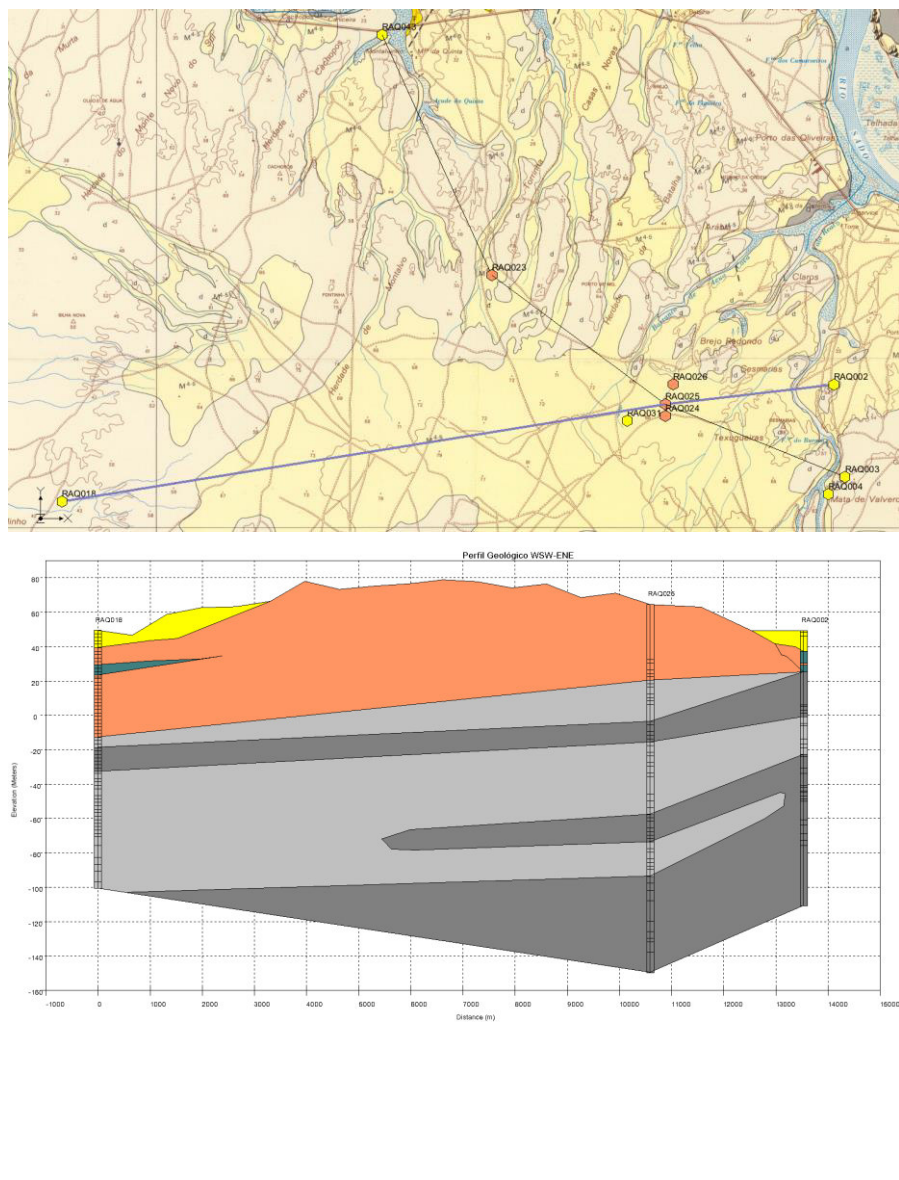
Figura 5.13 – Perfil geológico WSW-ENE entre as captações RAQ018, RAQ025 e RAQ002 constantes da base de dados da RioseAqüíferos e respectiva localização na Carta Geológica de Portugal à escala 1/50 000 Folha 39-C Alcácer do Sal
