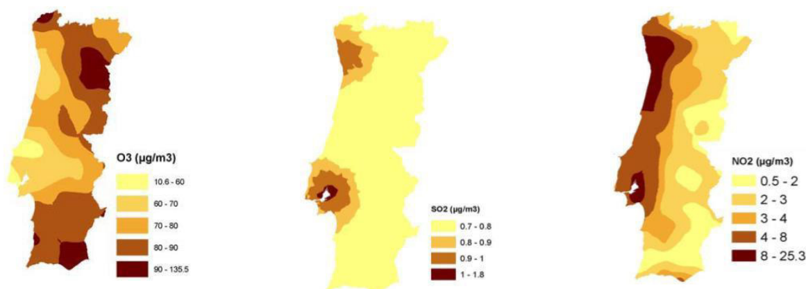
Figura 5.36 – Resultados das duas campanhas de avaliação da qualidade do ar – O 3 , SO 2 e NO 2
