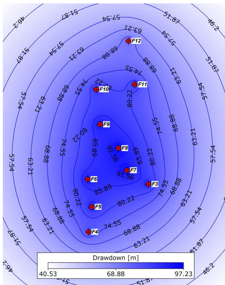
Figura 5.31 – Rebaixamento causado de extração de 10 L/s em contínuo durante 5 anos
