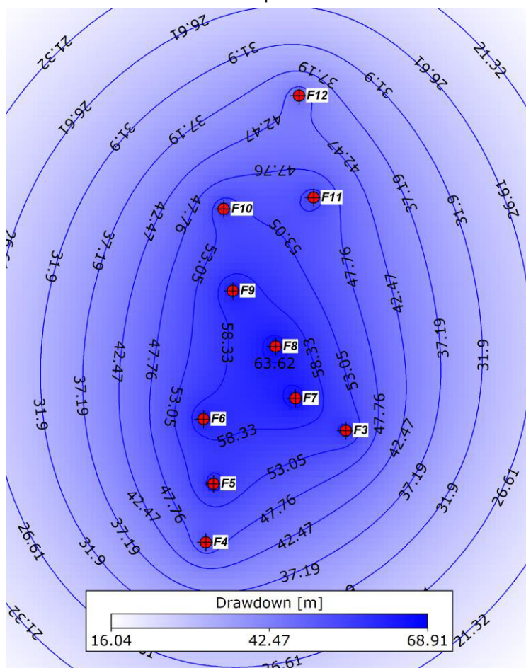
Figura 5.30 – Rebaixamento causado pela extração de 10 L/s em contínuo durante 365 dias
