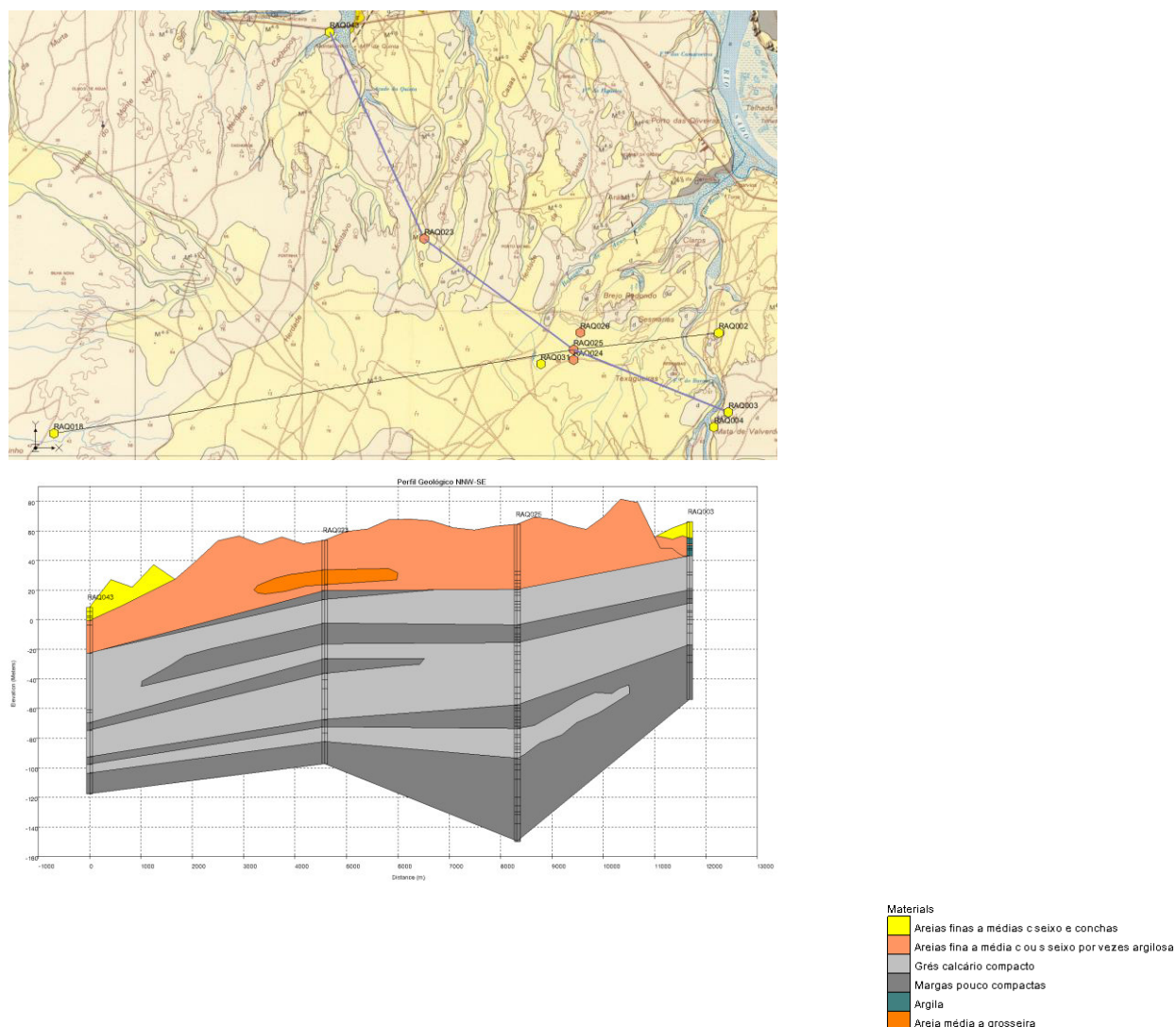
Figura 5.12 – Perfil geológico NNW-SE entre as captações RAQ043, RAQ023, RAQ025 e RAQ003 constantes da base de dados da RioseAquíferos e respectiva localização na Carta Geológica de Portugal à escala 1/50 000 Folha 39-C Alcácer do Sal
