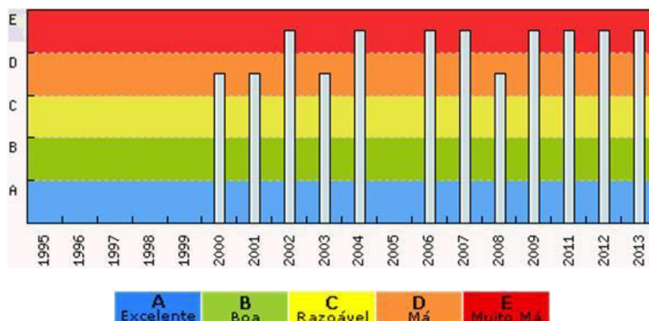
Figura 5.23 – Evolução da qualidade da água na estação 24G/02H (1995–2013)
