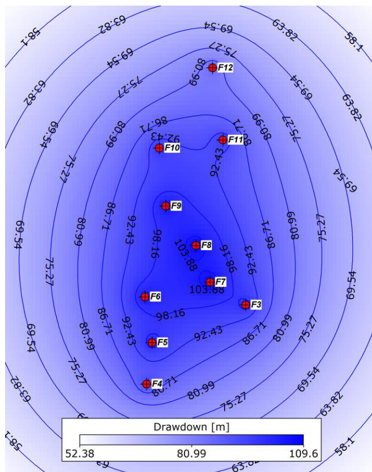
Figura 5.32 – Rebaixamento causado pela extração de 10 L/s em contínuo durante 10 anos
